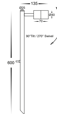
HV1423 Dimensions
