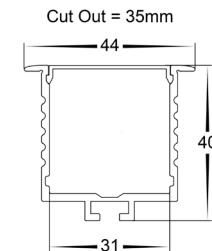
Dimensions
